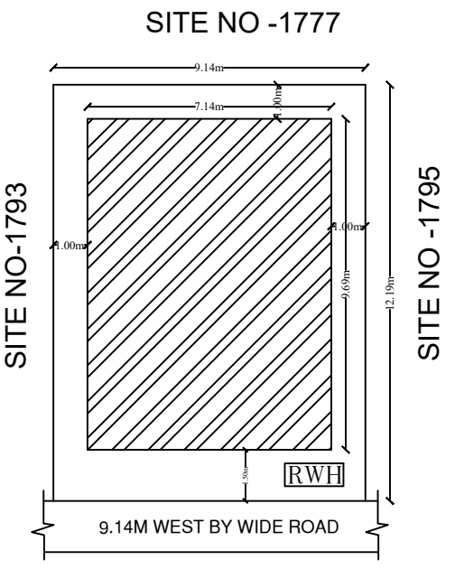
SITE PLAN (1:200)
